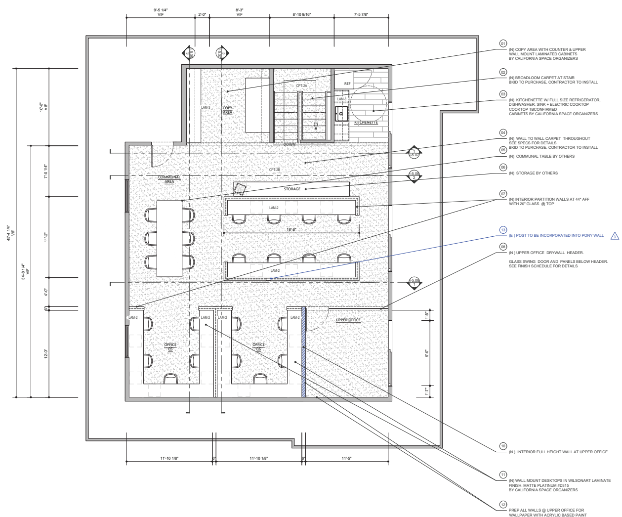
1 PLAN SCALE: 1/4"=1'-0"
